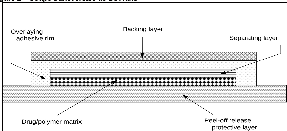
Figure 1 – Coupe transversale de BuTrans
